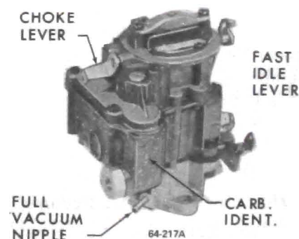
Figure 64-53 · Rochester MV Monojet Carburetor
