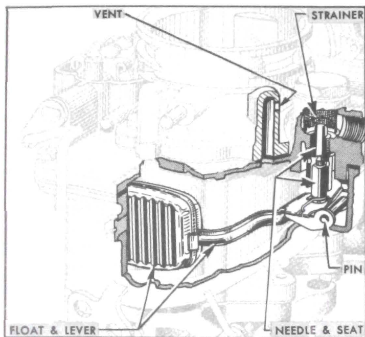
Figure 3-19—Float System—Carter WCD Carburetor
